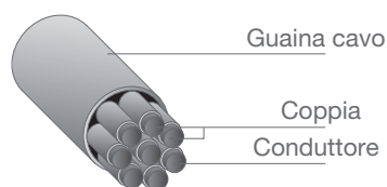
U/UTP
